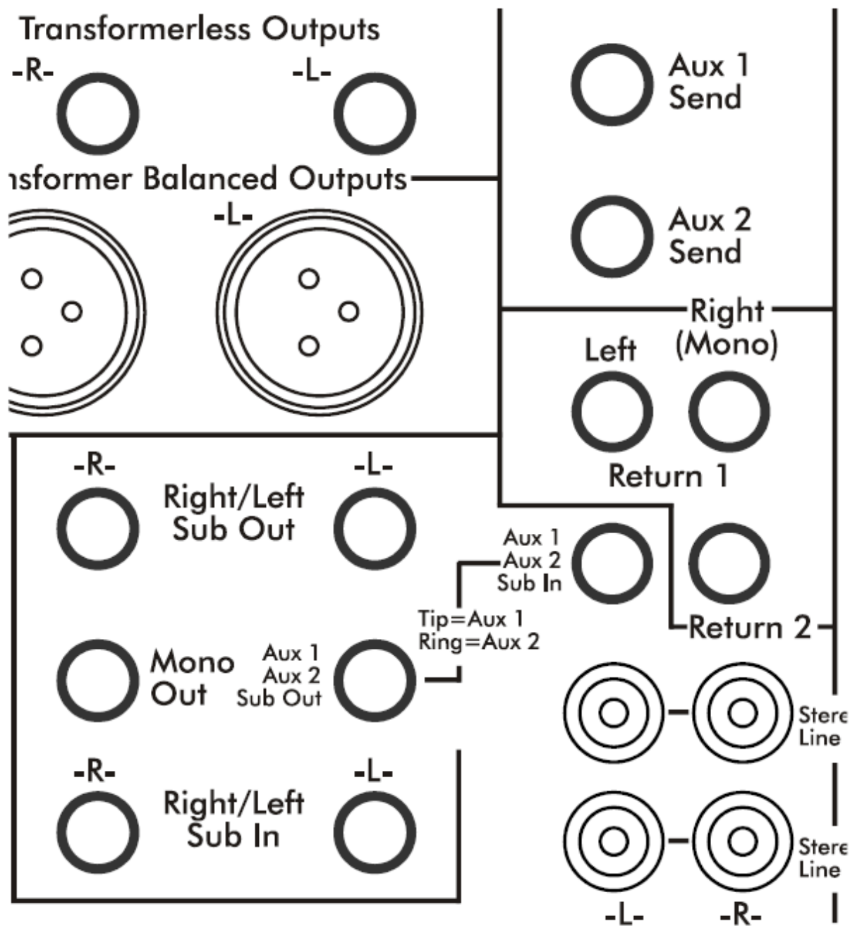
MX-508 の出力部分
